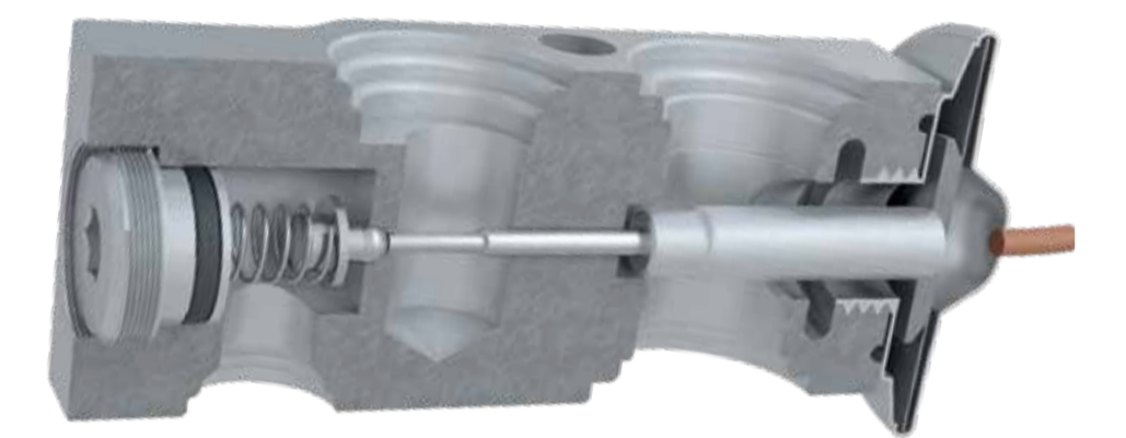
РАСШИРИТЕЛЬНЫЙ КЛАПАН
